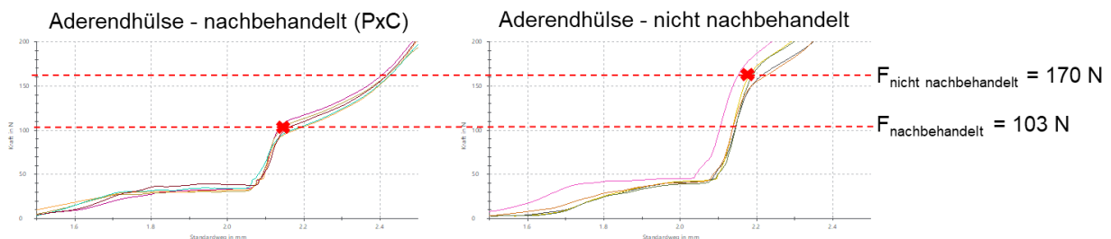
Abbildung 1: Kraft-Weg Diagramme beim Verpressen einer nachbehandelten (links) und einer nicht nachbehandelten Aderendhülse (rechts).
